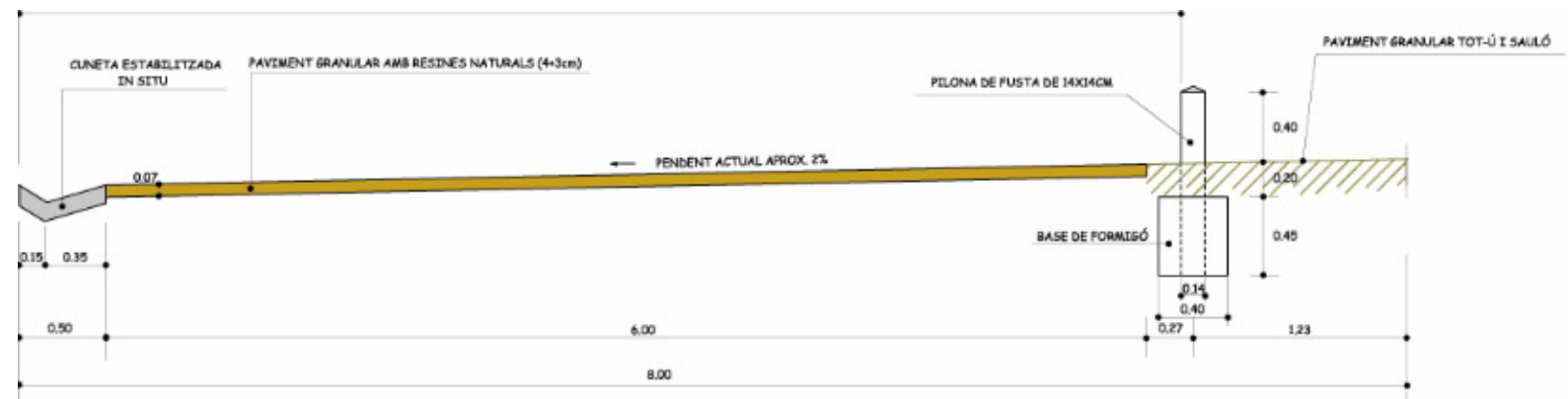
Secció tipus tram eixamplat
