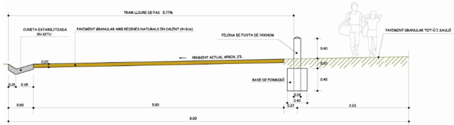
Secció tipus tram sense eixamplament
